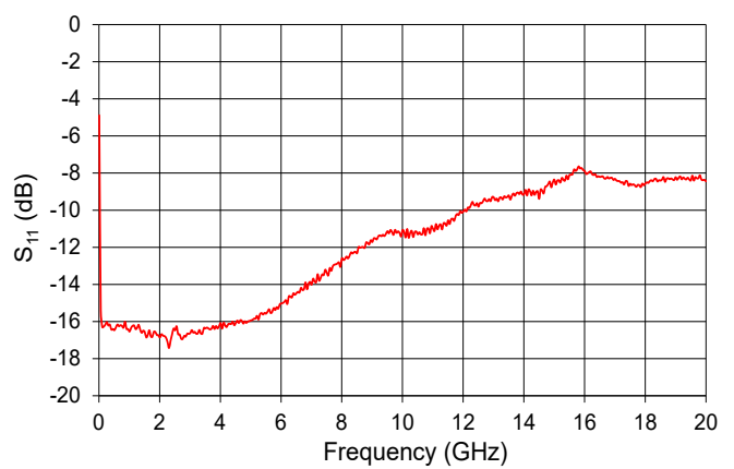
S_{11} Parameter Curve
